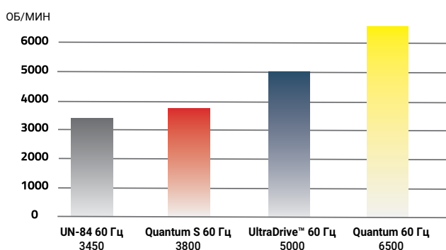
Сравнение частоты вращения двигателей
